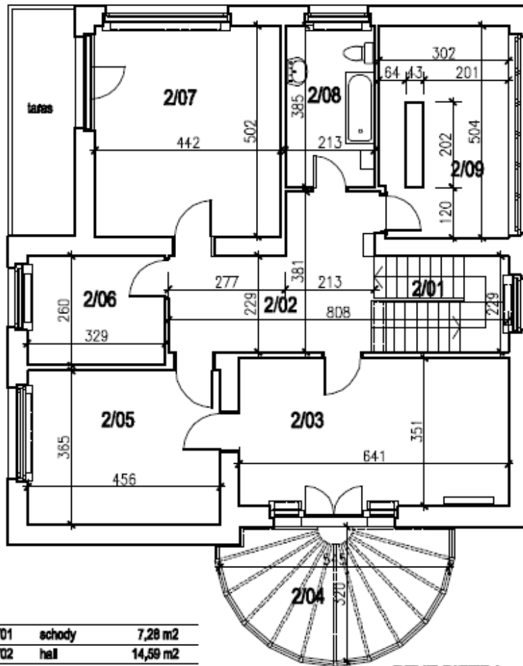
RZUT PIĘTRA
